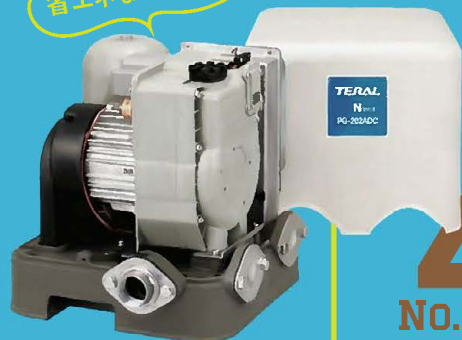
浅井戸用コンパクト式 インバーターポンプ PG-ADC
