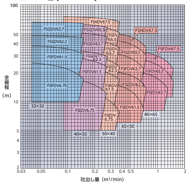
■ LPDV型 [3600min -1 ]
