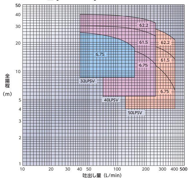
■ LPSV型 [3600min -1 ]
