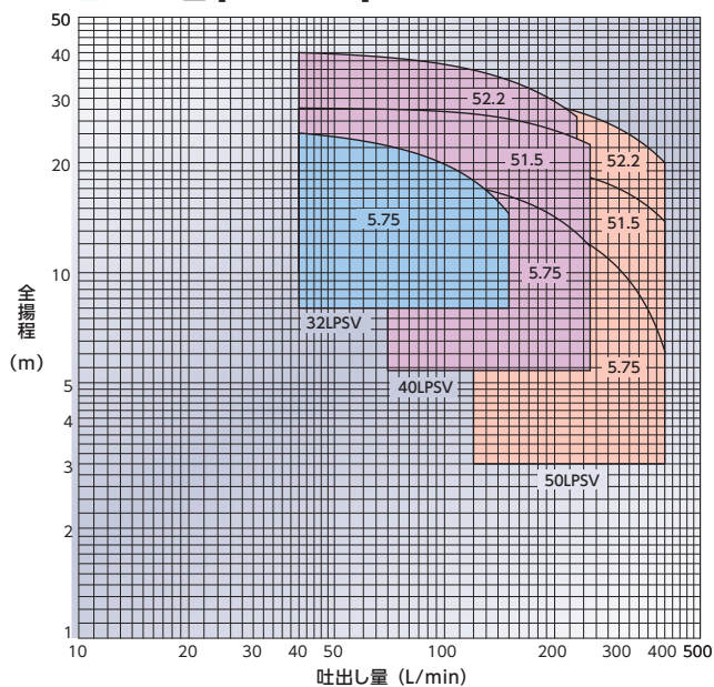
■ LPSV型 [3000min -1 ]
