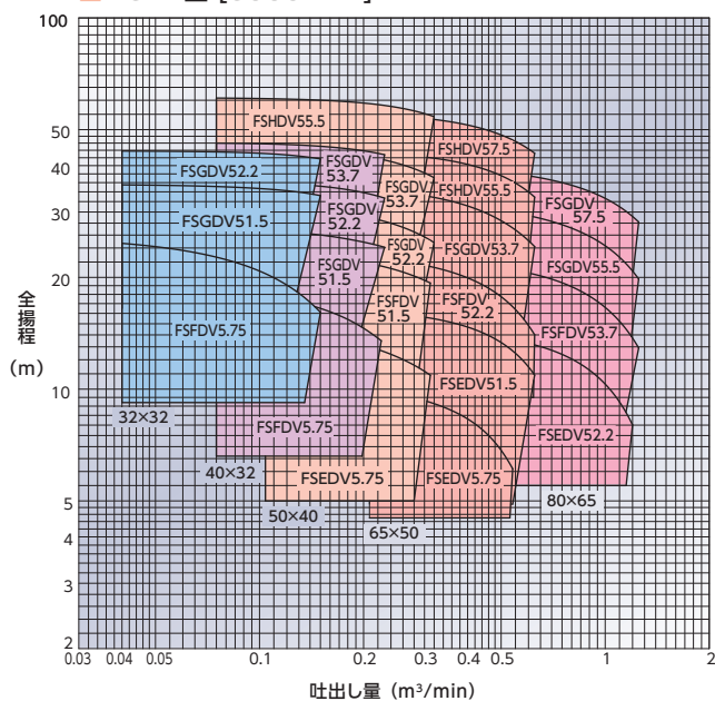
■ LPDV型 [3000min -1 ]
