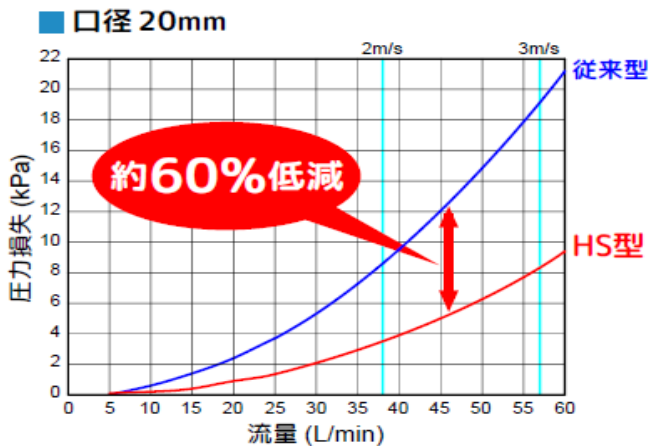
従来型とHS型の圧力損失比較表
